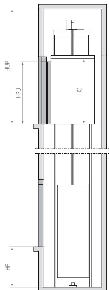
COUPE VERTICALE
